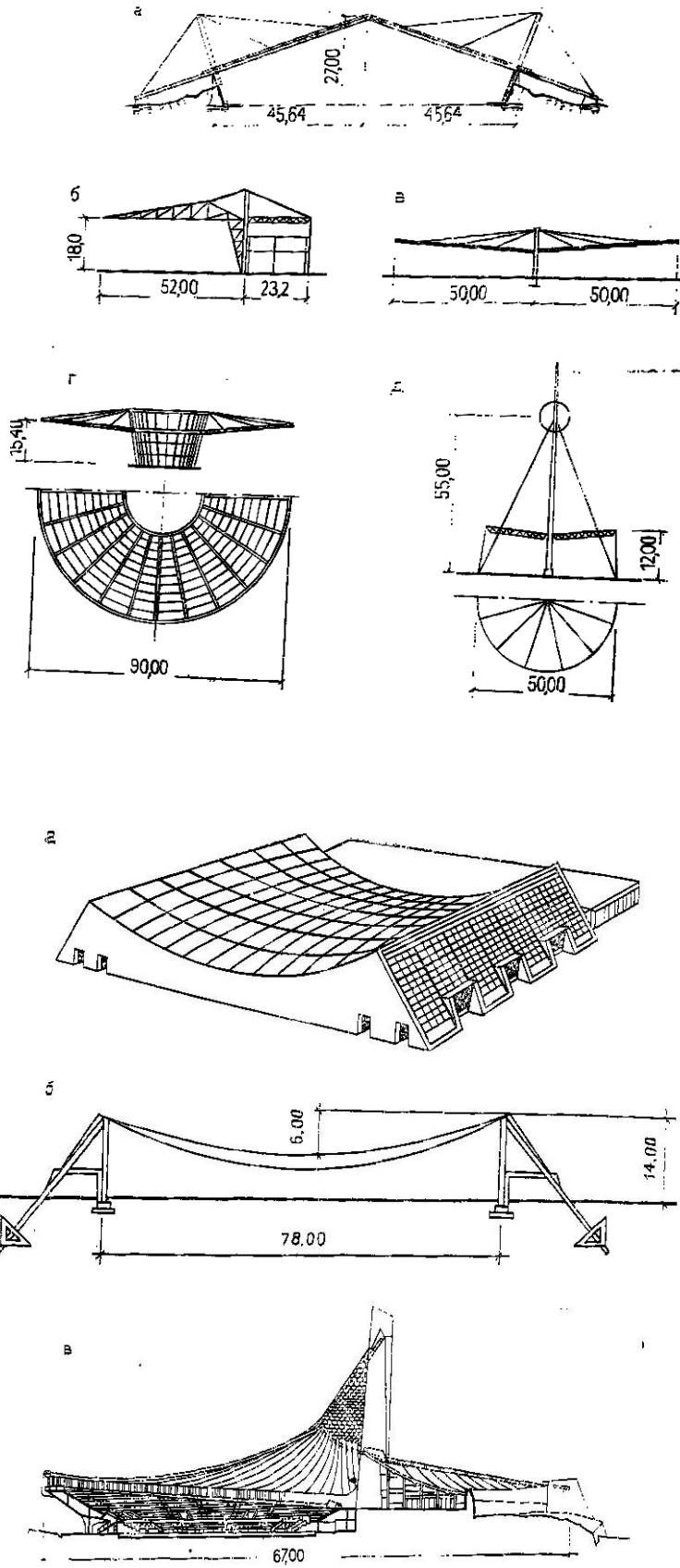
Рисунок 16. Консольно-подвесные покрытия; одноярусные висячие покрытия.
